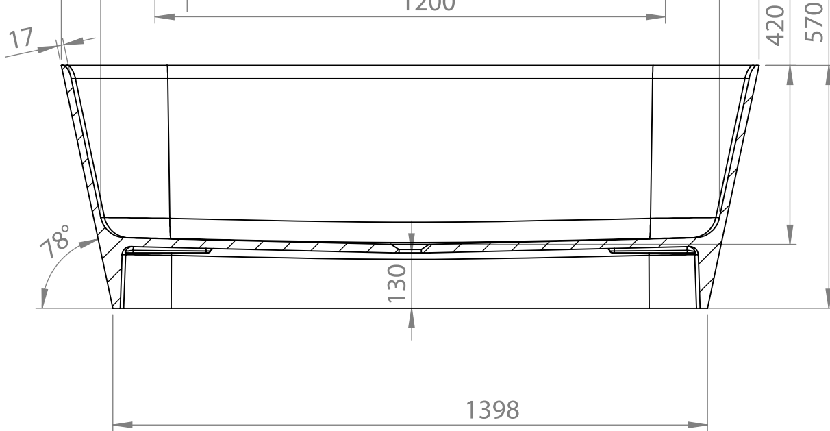
PRZEKRÓJ N-N SKALA 1 : 15
