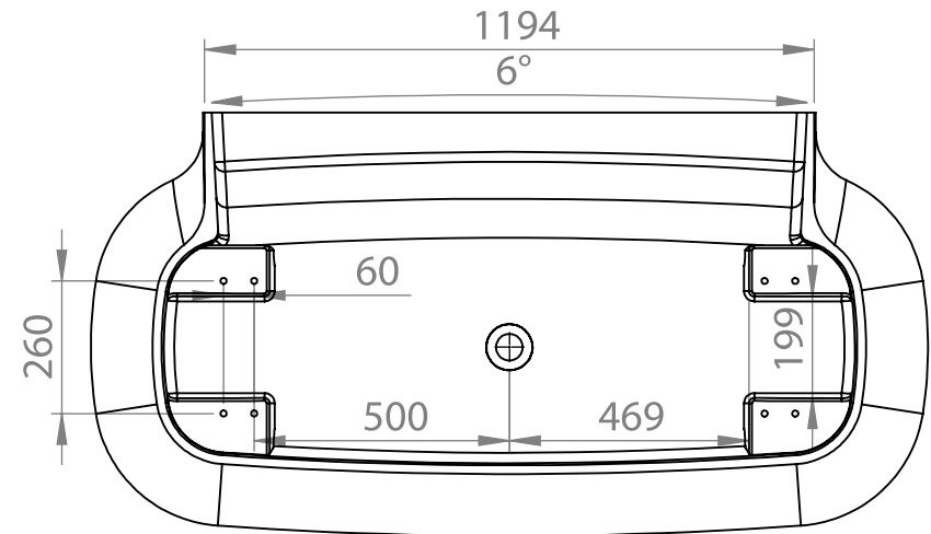
PRZEKRÓJ M-M SKALA 1 : 15
