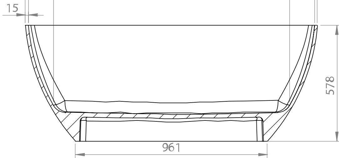
PRZEKRÓJ N-N SKALA 1:15
