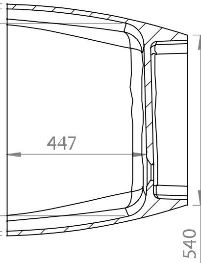
PRZEKRÓJ M-M SKALA 1:15
