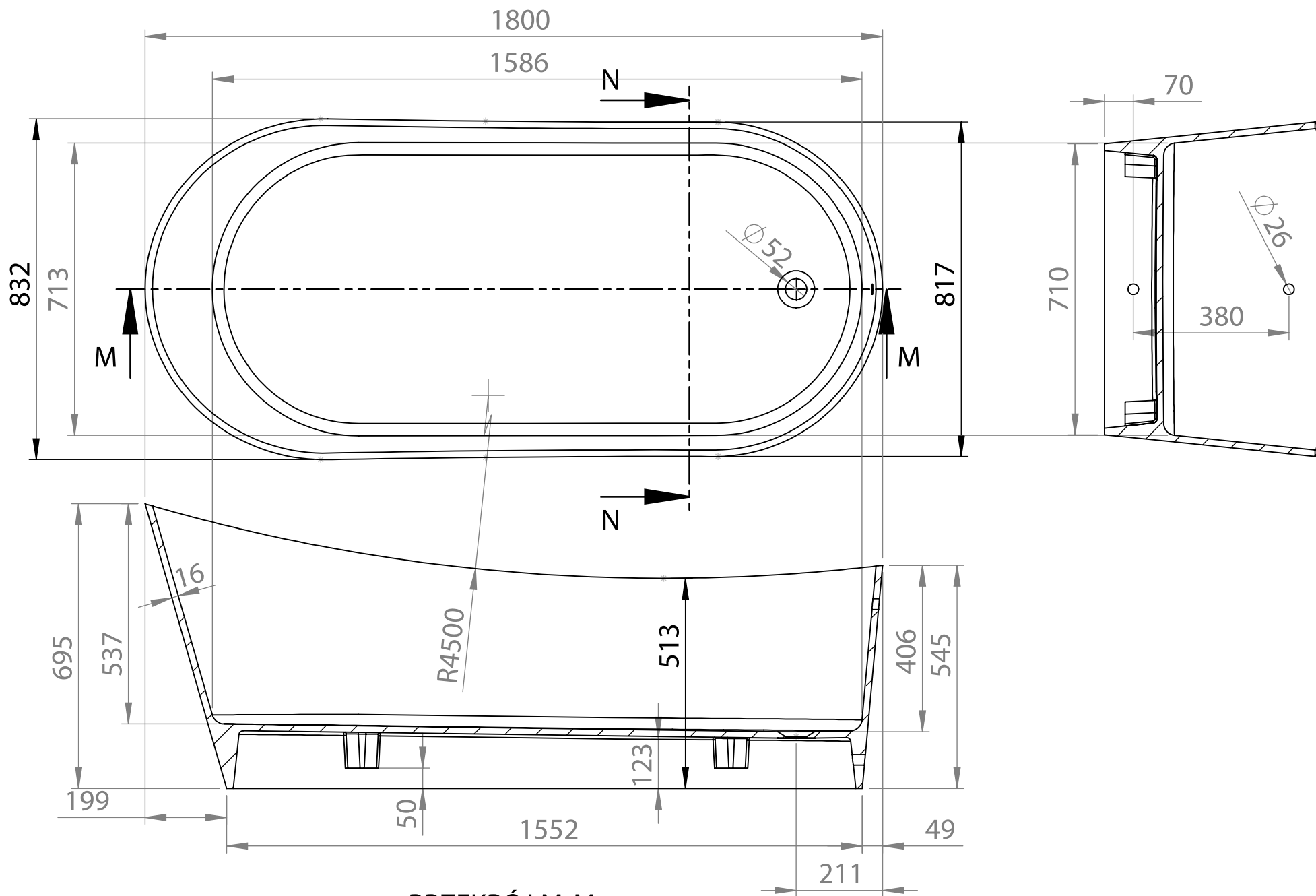
PRZEKRÓJ M-M SKALA 1 : 17
