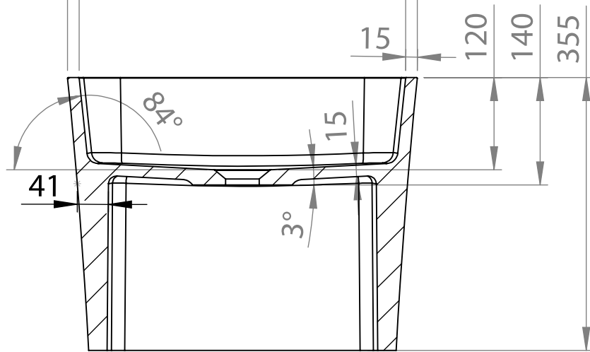
PRZEKRÓJ N-N SKALA 1 : 10
