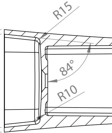
PRZEKRÓJ M-M SKALA 1 : 10
