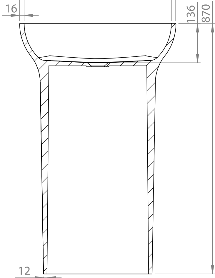
PRZEKRÓJ N-N
