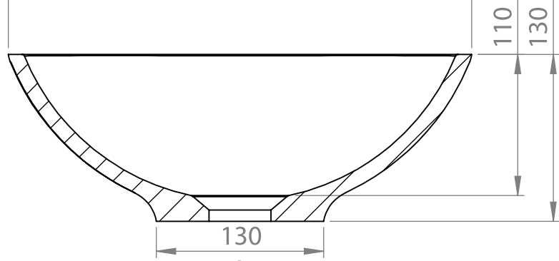
PRZEKRÓJ M-M SKALA 1 : 5
