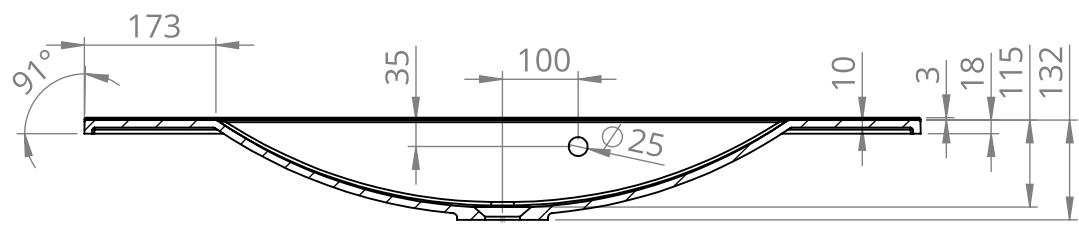
PRZEKRÓJ N-N
