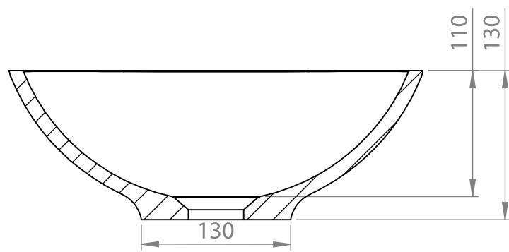
PRZEKRÓJ N-N SKALA 1 : 5
