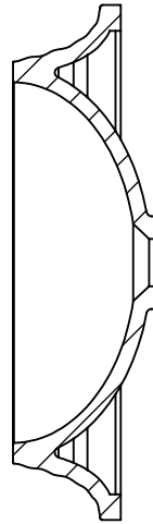
PRZEKRÓJ M-M SKALA 1 : 8
